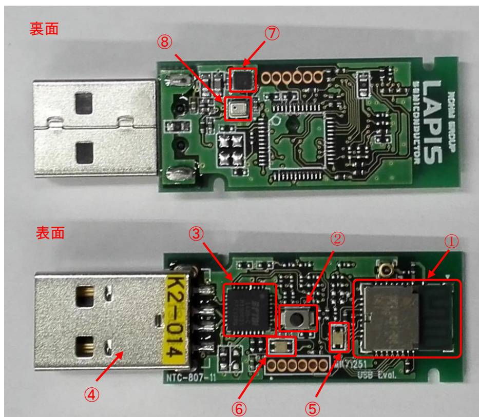
図 2-2 MK71251-02B USB ドングルの外観
